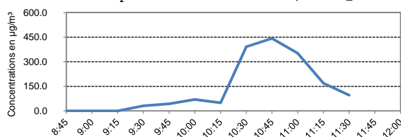
Moyennes horaires glissantes sur 15 min des concentrations en SO 2 à Montravel le 07 novembre 2019, DSI 2019_007
